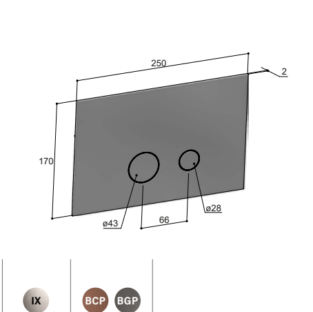
Actuator plate for Geberit Sigma 8 - Sigma 12, with magnetic fixing Placca di comando per Geberit Sigma 8 - Sigma 12, con fissaggio magnetico Plaque de déclenchement pour Geberit Sigma 8 - Sigma 12, avec fixation magnétique Drückerplatte für Geberit Sigma 8 - Sigma 12, mit magnetischer Befestigung Placa de acionamento para Geberit Sigma 8 - Sigma 22, con fijación magnética
